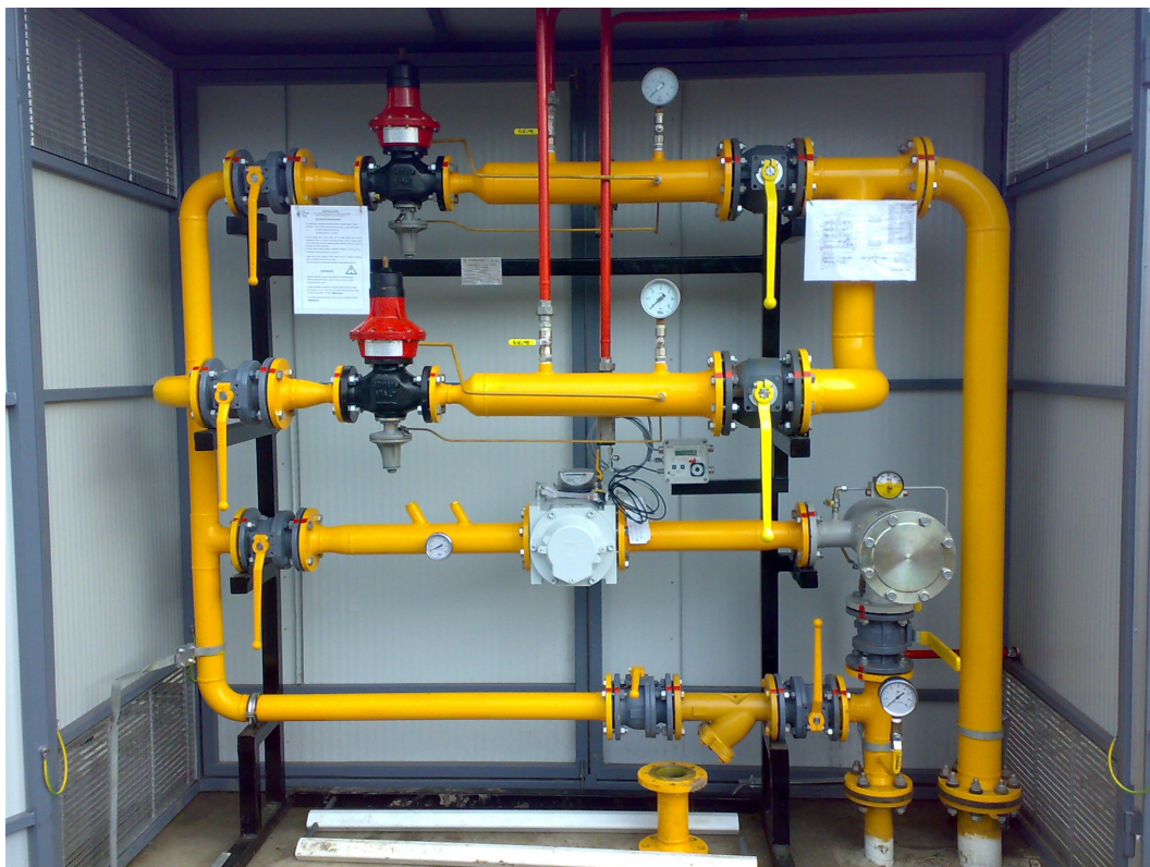
ALLTECH FERMIN - Senta Merno-regulaciona stanica za prirodni gas - 1.200 m 3 /h
